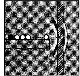
図1 受振点1個、震源30個で、トンネル \perp 反射面である破碎帯様の反射面を探索
