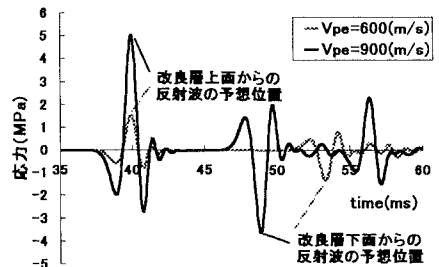
図-3 改良層の速度変化に伴う反射波形変化
