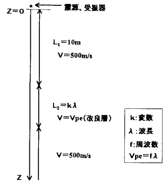
図-1 地盤改良後想定モデル
