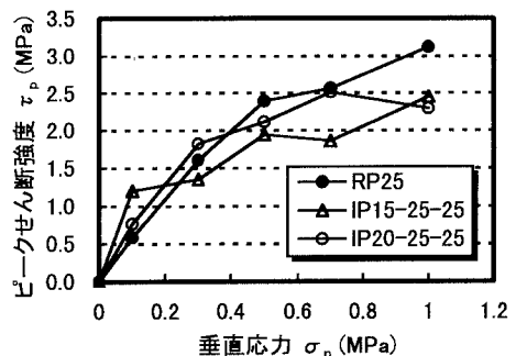
図-2 各供試体の破壊包絡線
