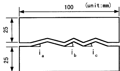
図-1 石膏供試体側面図
