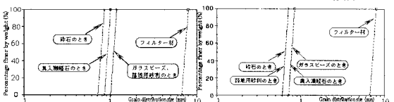
図-5 (1) 緩詰め (2) 密詰め 各フィルター材に対する地山砂の目詰まりしない限界粒度
