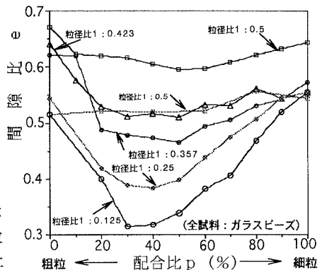
図-6 粒径比による間隙比の変化
