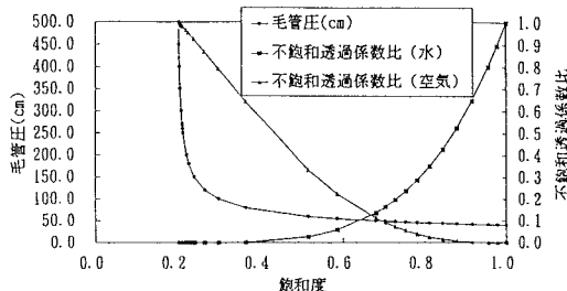
図-2 水分特性曲線 ( \lambda = 2.3 , S_r = 0.2 )
