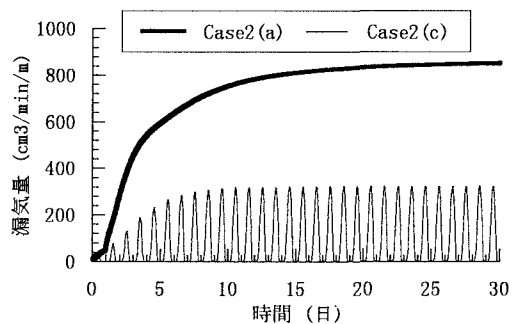
図-6 単位時間あたりの漏気量の時間変化(Case2(c))
