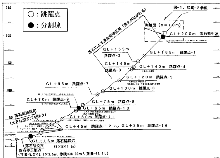
図-1 落石経路断面図
