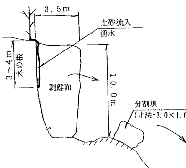
図-2 落石発生源の模式図
