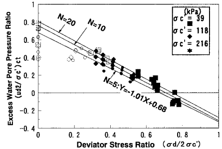
図-2 繰返し三軸試験による偏差応力比と偏差応力に伴う過剰間隙水圧比の関係
