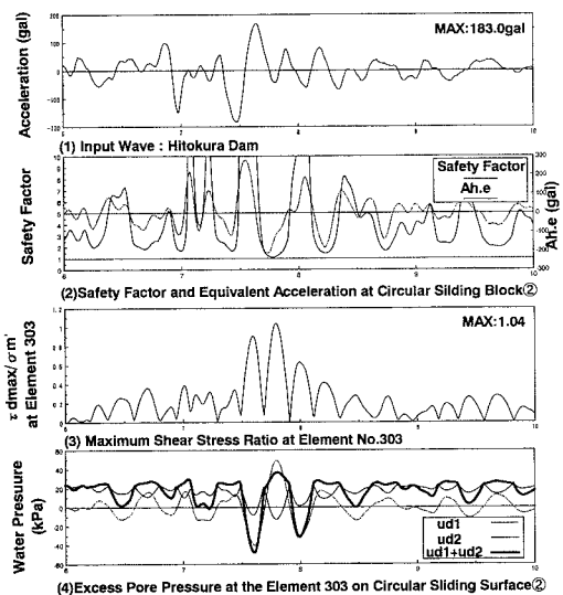
図-4 すべり安全率、等価瞬間加速度、最大せん断力比、および過剰間隙水圧の時刻歴(CASE2, 円弧②)
