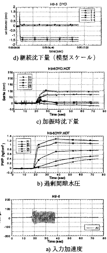
図-3 4脚対策模型の実験結果
