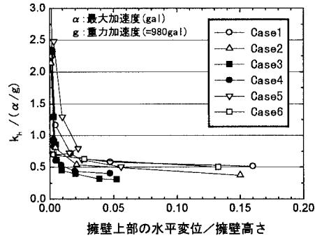
図-4 擁壁の水平変位と水平震度／最大加速度の関係
