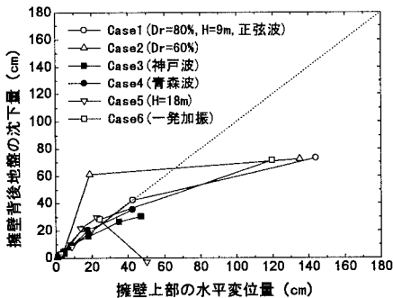
図-3 擁壁の水平変位量と背後地盤の沈下量の関係
