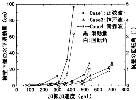
図-2 加振加速度と擁壁の変位の関係
