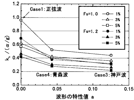
図-5 波形の特性値と水平震度／最大加速度の関係
