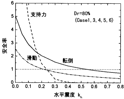
図-1 水平震度と安全率の関係
