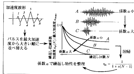
図-6 波形の特性値aの概要 5)
