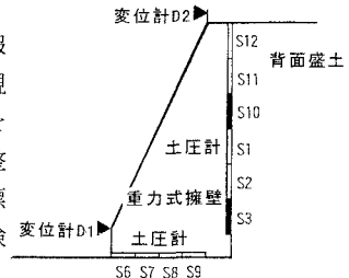
図-1 実験模型断面
