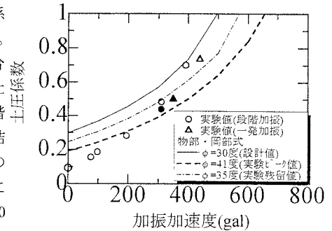
図-3 加振加速度と土圧係数の関係（正弦波加振）
