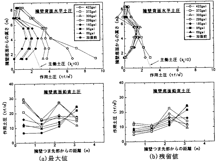
図-5 加振中の土圧分布 (Case1)
