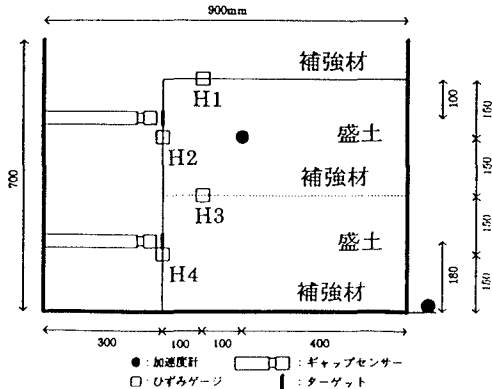
図-1 盛土と計測装置
