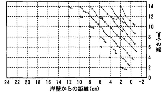
(c) ケース S-H1 (静的実験, h=15\text{cm} , fast)
