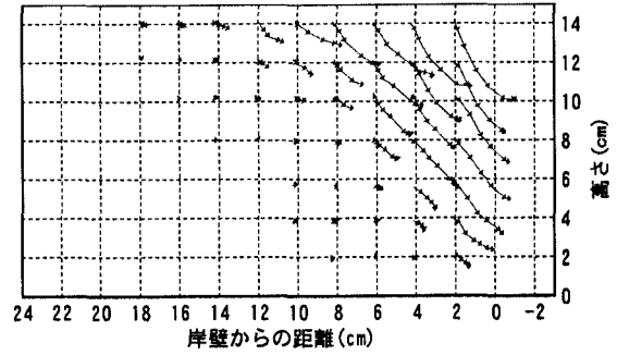
(a) ケース D-H3 (動的実験, h=15\text{cm} , fast)
