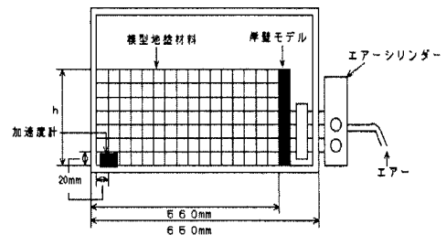
図 2.1 実験モデル
