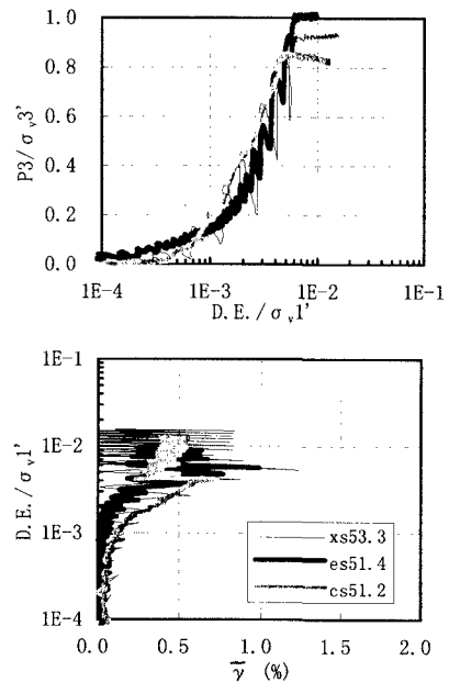
図2 液状化振動台実験結果
