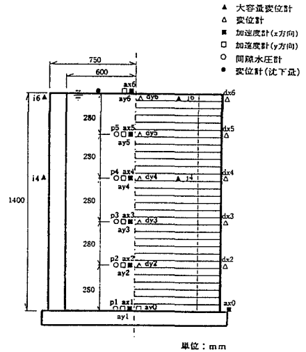
図1 せん断土槽の模式図
