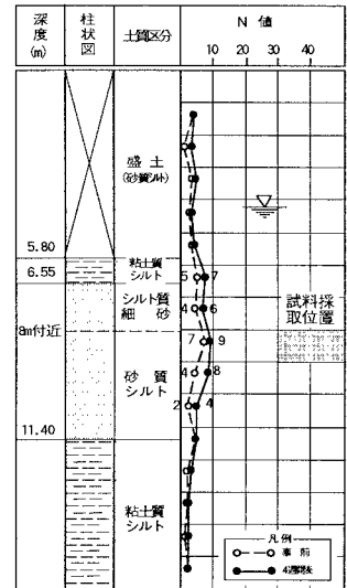
図-2 N値の分布
