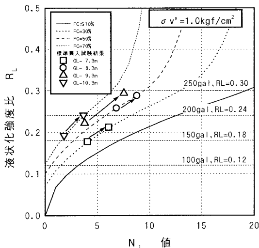
図-3 推定液状化強度比 R_L ~ N_1 値の関係
