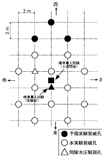
図-1 標準貫入試験位置
