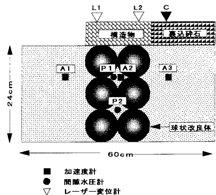
図一 実験概要図
