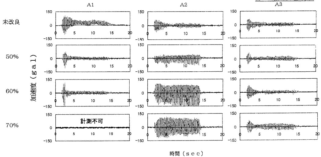
図-4 A1～A3での応答加速度
