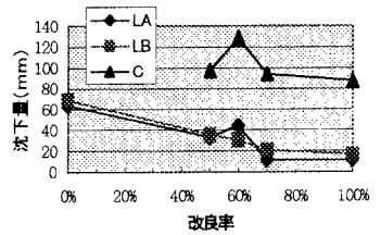
図-3 最大沈下量比較図
