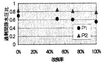
図-2 最大過剰間隙水圧比比較図
