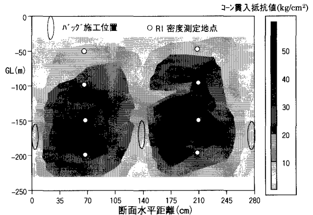
図-4 a-a'断面の施工後コーン貫入抵抗値
