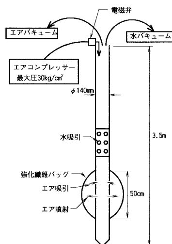
図-1 施工ツールの概要
