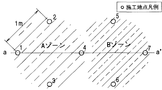
図-3 施工地点の平面図
