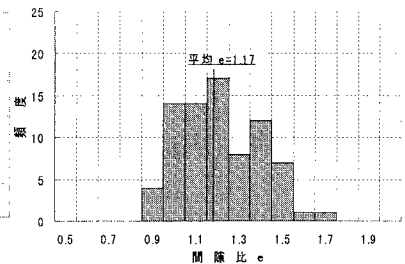
図-4 C地点の間隙比のヒストグラム
