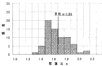
図-3 B地点の間隙比のヒストグラム
