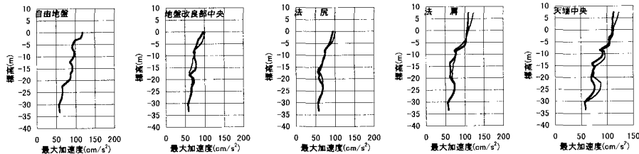
図-7 地盤改良を行った場合と行っていない場合との最大加速度の深度分布の比較(細線:未改良、太線:改良)
