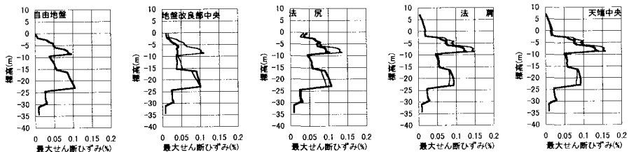
図-6 地盤改良を行った場合と行っていない場合との最大せん断ひずみの深度分布の比較(細線:未改良、太線:改良)
