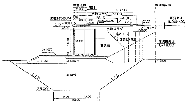
図2 六甲アイランドにおいて背後地盤が改良されていた護岸の例 5)
