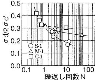
図-6 DA=1%における繰返し回数と繰返しせん断応力比の関係
