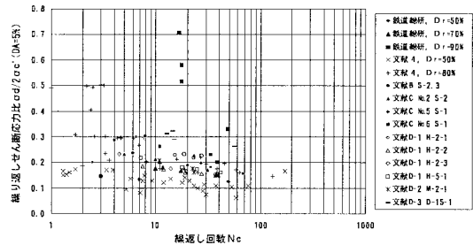
図1 繰返し回数と応力比の関係
