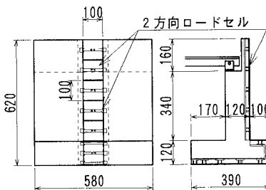
圖 2 模型橋台
