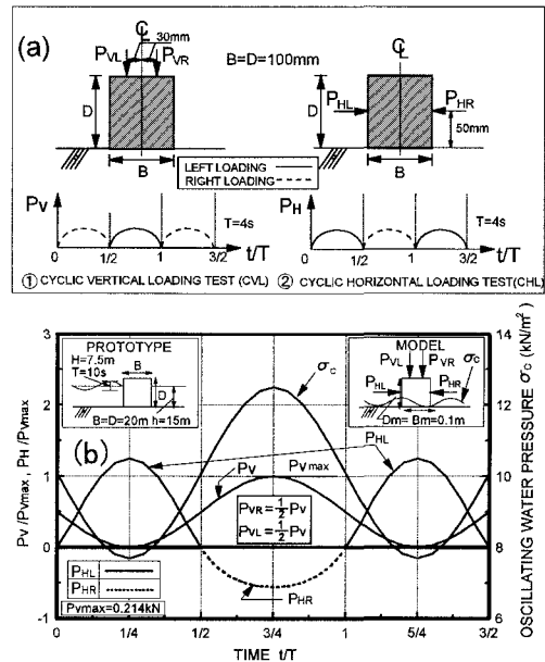
図-1 試験の載荷方法
