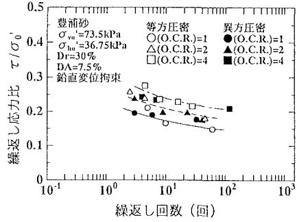
図3 繰返し応力比と繰返し回数の関係 （圧密方法の影響）
