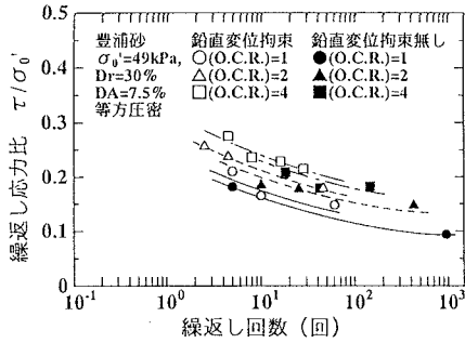
図2 繰返し応力比と繰返し回数の関係 （鉛直変位拘束の影響）
