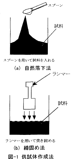
図-1 供試体作成法
