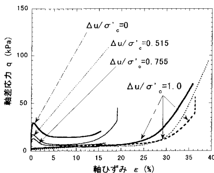
図-2 応力～ひずみ関係(自然落下法)
