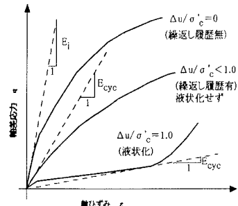
図-4 変形係数の定義
