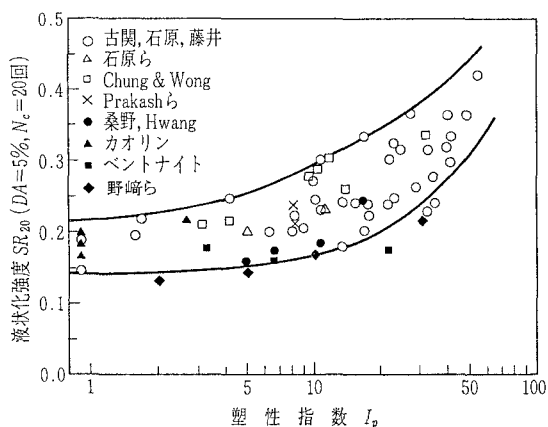
図 4 塑性指数と液状化強度の関係
