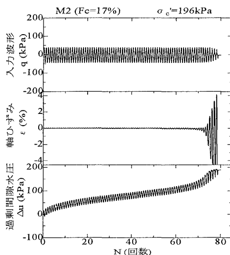
図 2 繰返しせん断試験結果 \sigma'_{cv}=196\text{kPa}
