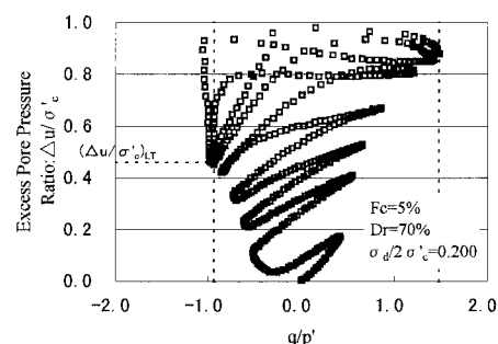
図-4 \Delta u/\sigma'_c と q/p' の関係
