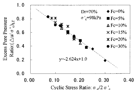
図-5 過剰間隙水圧と応力比の関係
