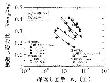
図4 R~Nc関係
