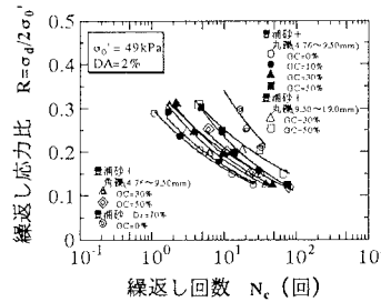
図3 R~Nc関係
