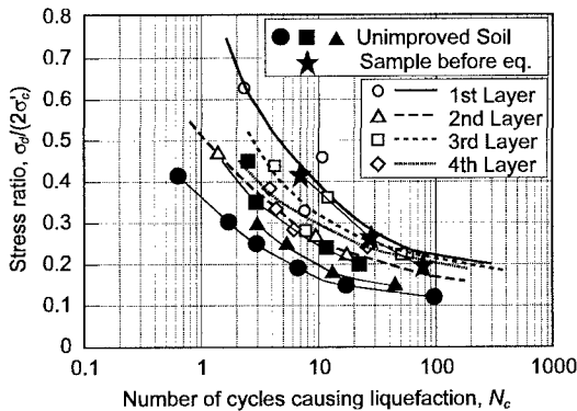
図-4 既往の研究との比較（DA=5%）
