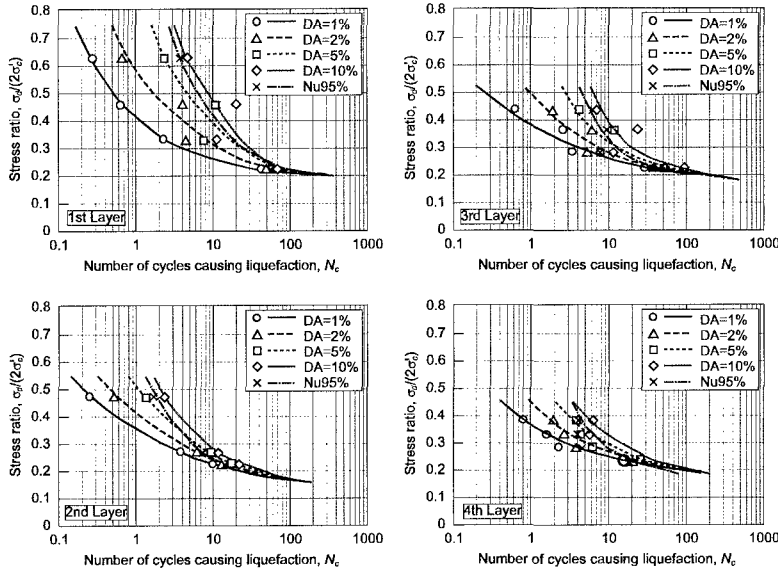
図-3 繰返しせん断応力比と繰返し数の関係
