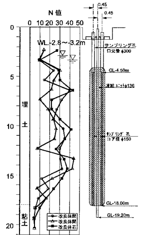
図-1 柱状図と試料採取位置
