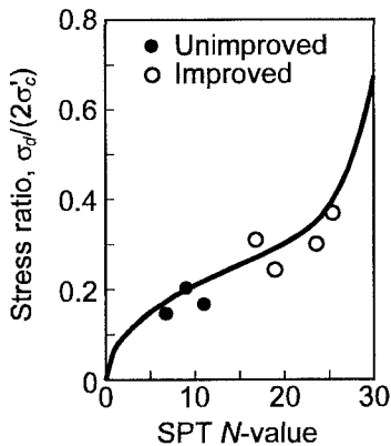
図-5 簡易法との比較（ D_{50}=2.5\text{mm} , F_c=8\% として計算． \sigma'_v = 1\text{kg/cm}^2 ）
