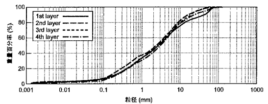
図-2 平均粒度分布
