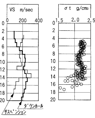
図-5 S波速度 図-6 湿潤密度
