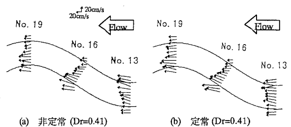
図4 60.0 (l/sec) の表面流速分布形の比較
