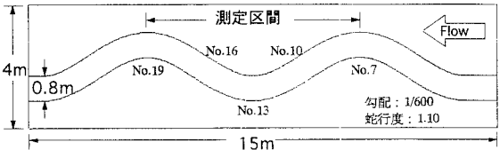
図1 実験水路平面図
