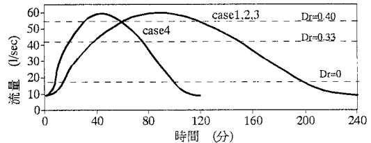
図2 設定ハイドログラフ
