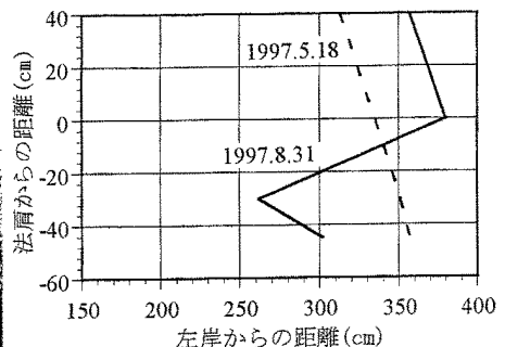
図-3 横断形状 (A-A')
