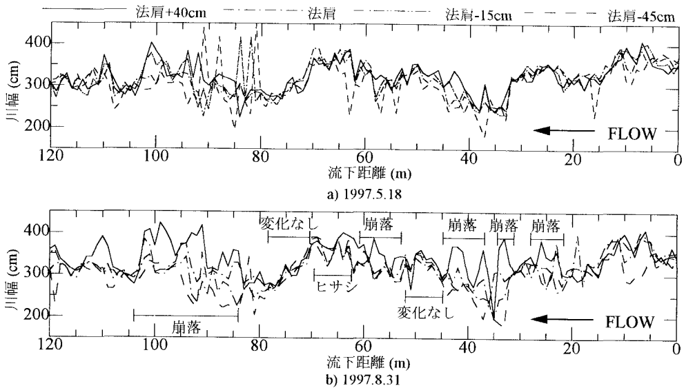
図-4 河岸の縦断形状
