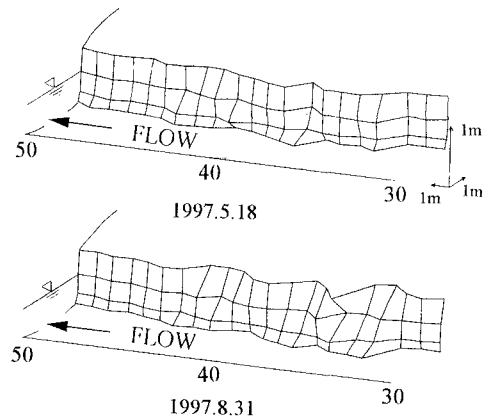
図-5 30～50m の区間の河岸形状
