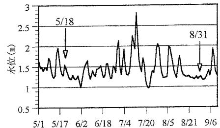
図-2 洪水による水位の変化
