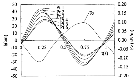
図3 変動間隙水圧(h)および変動流体力( F_z )
