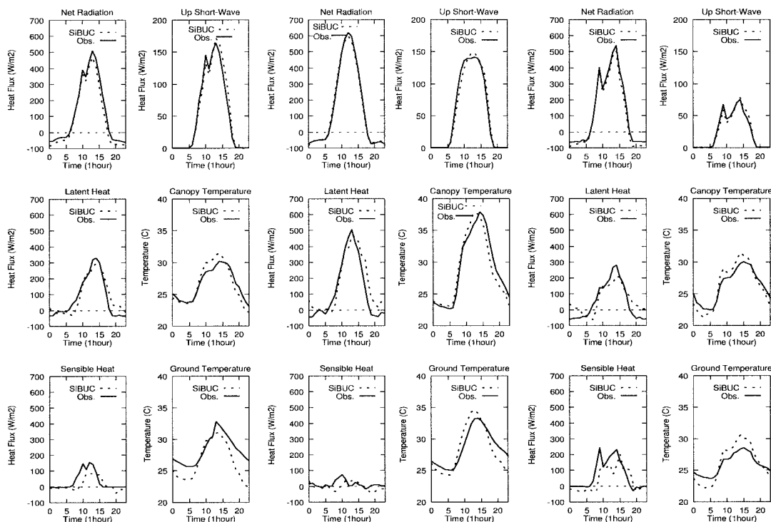
図1 SiBUCと観測の比較(畑地)
