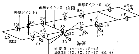
図-2 測点配置図
