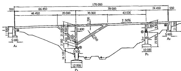
図-1 一般図
