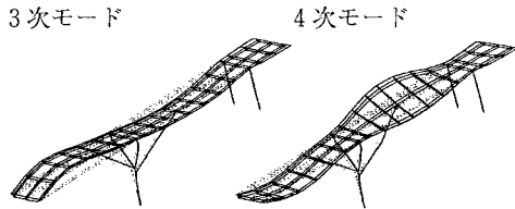
図-4 振動モード図
