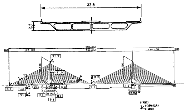
図-1 構造一般図、地震計設置位置
