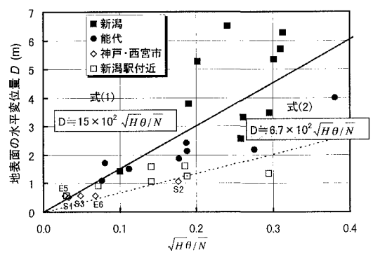
図 5 地表面変位量と \sqrt{H\theta}/\bar{N} の関係
