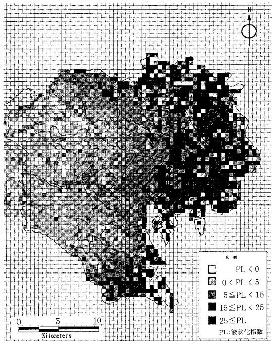
図-2 液状化指数(PL値)分布(type II)
