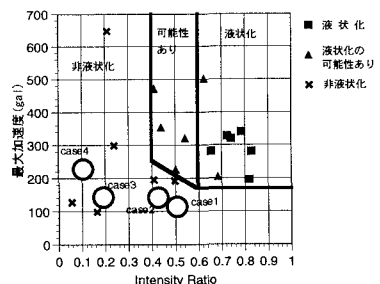
図-10 Intensity 比と最大加速度値の関係
