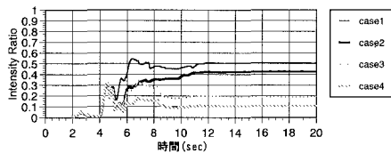
図-7 Intensity比の時刻歴
