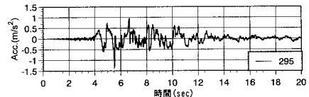
図-3 入力地震動
