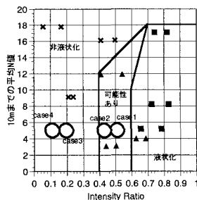
図-8 Intensity 比と平均 N 値の関係
