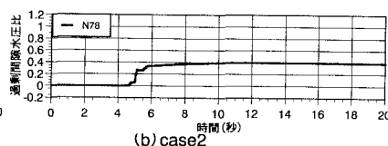
図-5 過剰間隙水圧比の時刻歴
