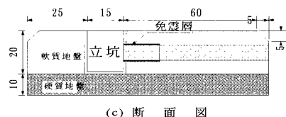
(c) 断面図
