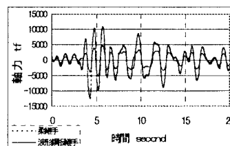
図 9 要素 20 の軸力の時刻歴
