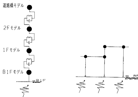
図-3：Step-2 モデル
