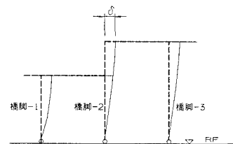
図-6：橋脚の応答解析模式図（Step-3）
