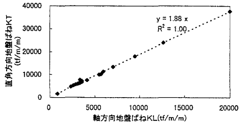
図-5 軸直角方向に対する地盤ばね定数
