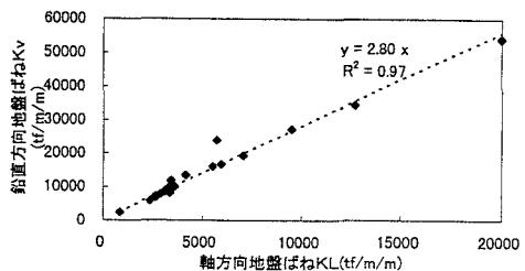
図-6 鉛直方向に対する地盤ばね定数
