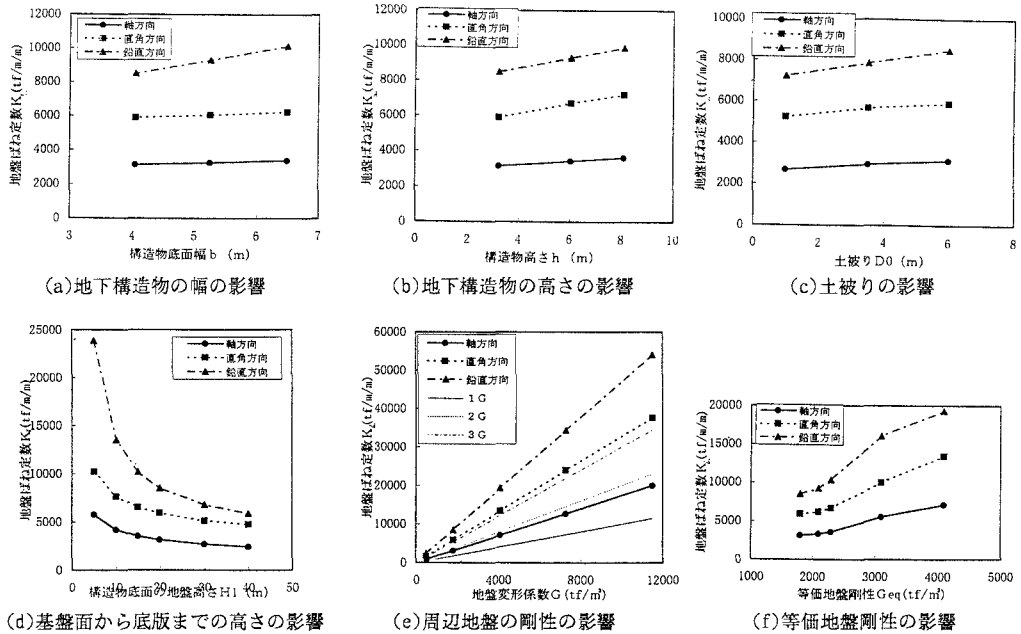
図-2 各パラメータと軸方向地盤ばね定数 K_L との関係
