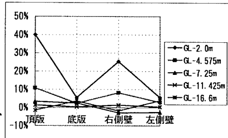
図-4 曲げモーメントの差の割合 \{ (M-\phi) - (Fiber) \} / (Fiber)
