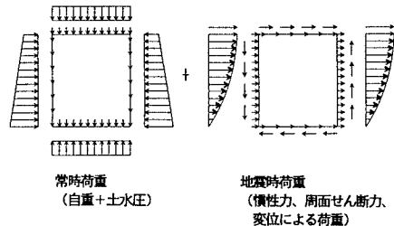
図-3 荷重図
