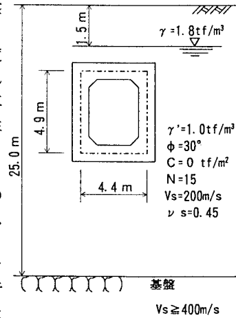
図-1 検討断面図
