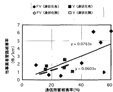
図3.1 他事業者管路との被害率比較
