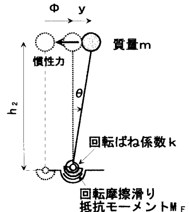
図 5 継手より上部の一自由度系モデル
