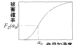
図1 被害曲線
