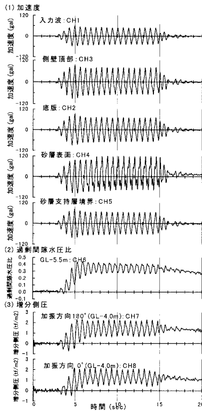
図-4 応答波形（入力加速度：58gal）
