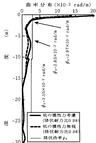
図-4 杭に生じる曲率分布 (Ⅲ種地盤)
