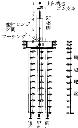
図-1 桁一橋脚一杭基礎系の解析モデル
